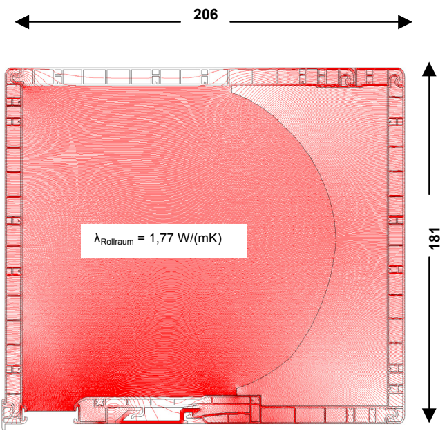
Rollladenkasten 181, Rev. hinten Verlauf der Wärmestromlinien
